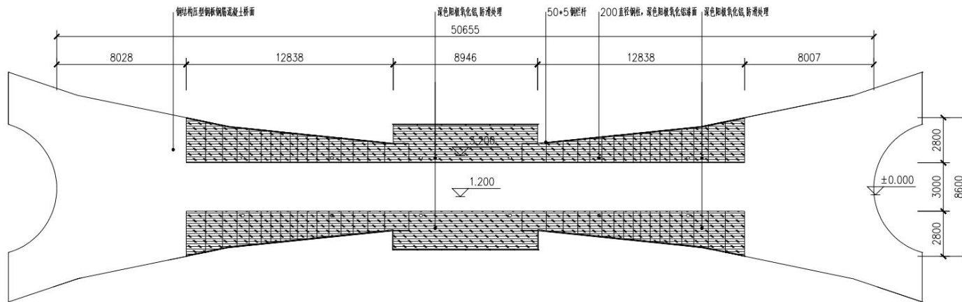
平面图
